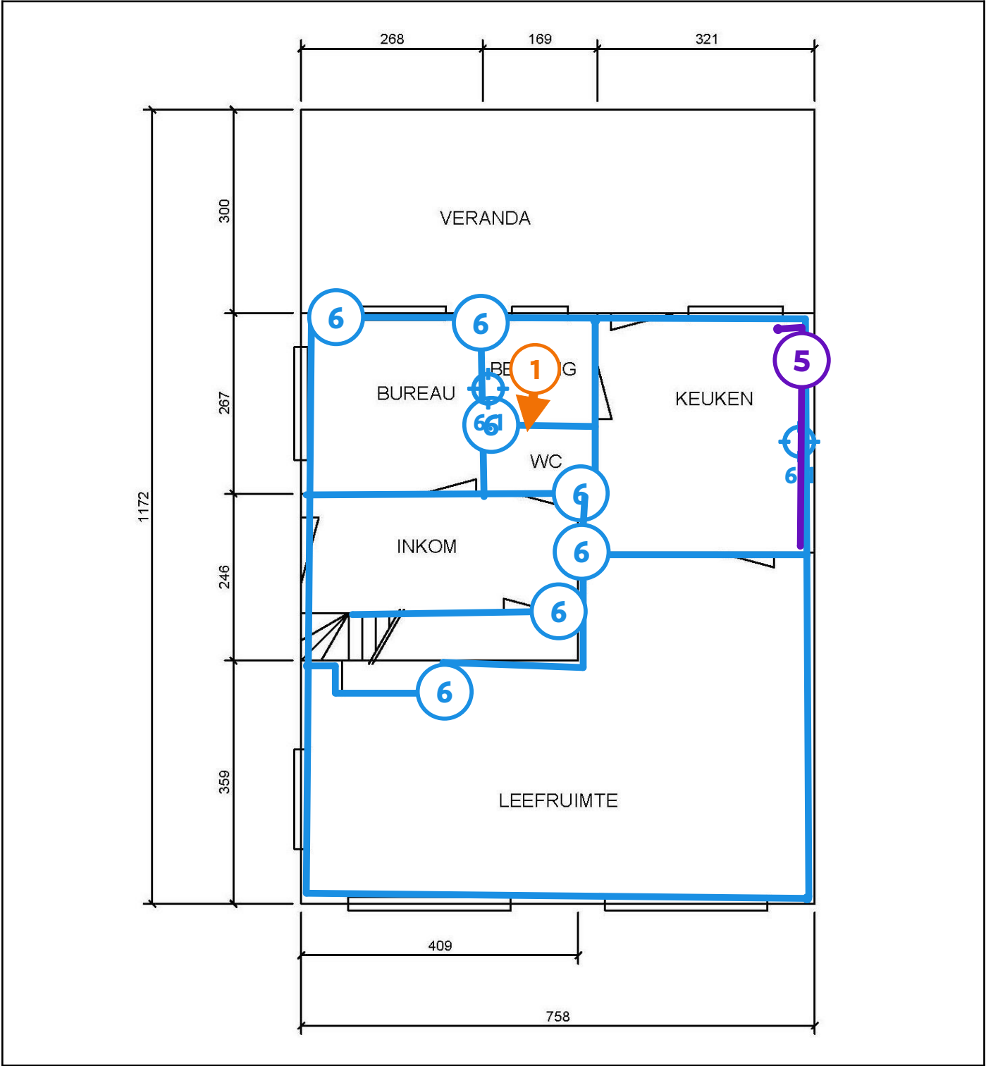
Legende van plan 1.1: PLAN_Sierheesterlaan 13_GV
